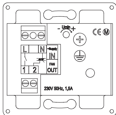
Circuito impreso
